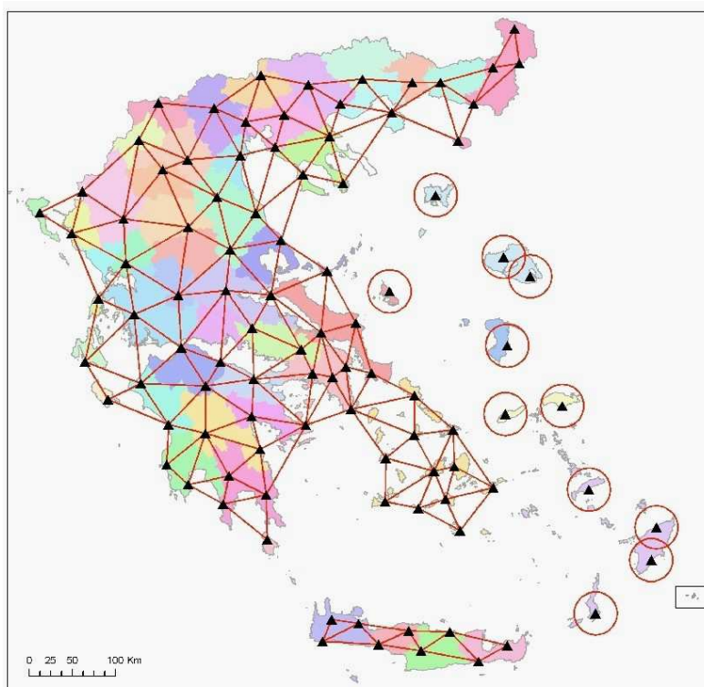
Εικόνα 1: Οι θέσεις των 98 Σταθμών Αναφοράς του HEPOS.
